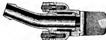
Fig. 2994. Longitudinal Section.
